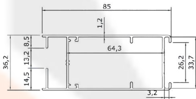
8343 ENCUENTRO/TAPA CANTO DE 25MM Peso: 0,290kg/m
