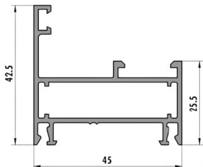
8216 MARCO UNIVERSAL Peso: 0,726kg/m
