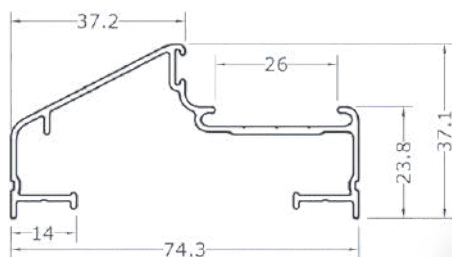
8078 PARANTE PUERTA 90° Peso: 0,897kg/m
