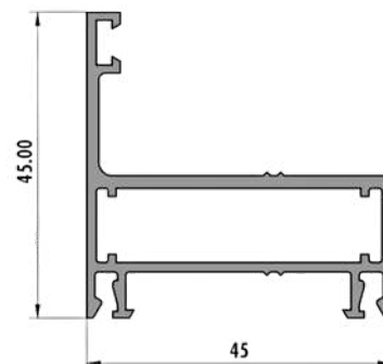
8259 MARCO DESPLAZABLE Peso: 0,726kg/m
